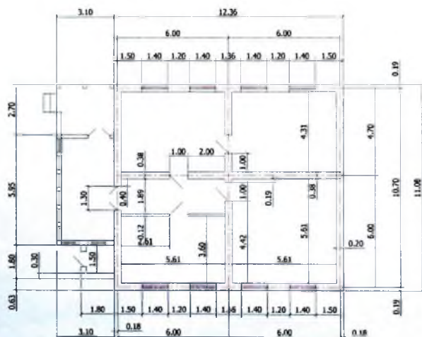
План фундамента
